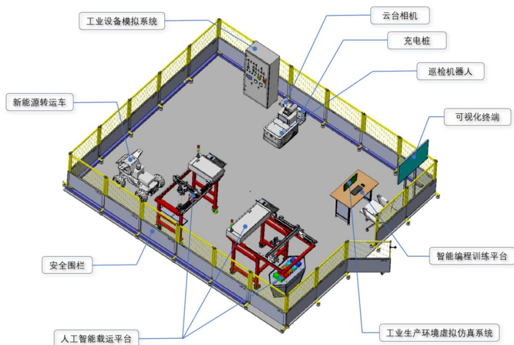
图1 人工智能工业应用平台布局示意图(职工组)
