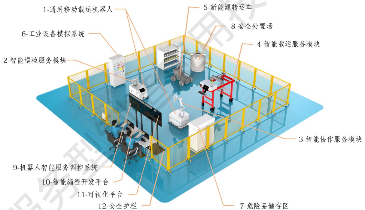
图 1 职工组（含教师）机器人智能服务与应用系统平台结构图
