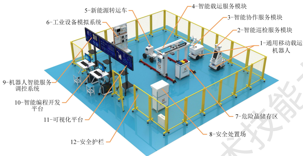
图 2 学生组机器人智能服务与应用系统平台结构图
