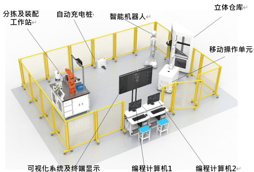
图 1 职工组工业机器人人工智能技术应用平台总布局示意图
