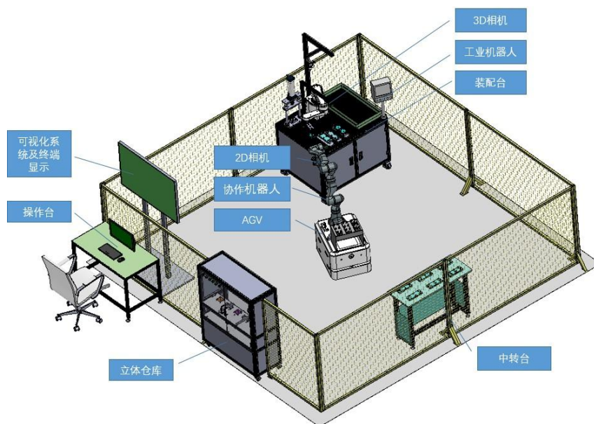
图 2 学生组工业机器人人工智能技术应用平台总布局示意图
