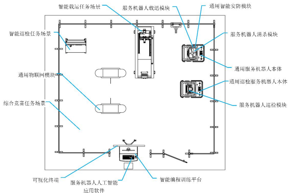
图 4 服务机器人人工智能技术应用平台俯视图（学生组）
