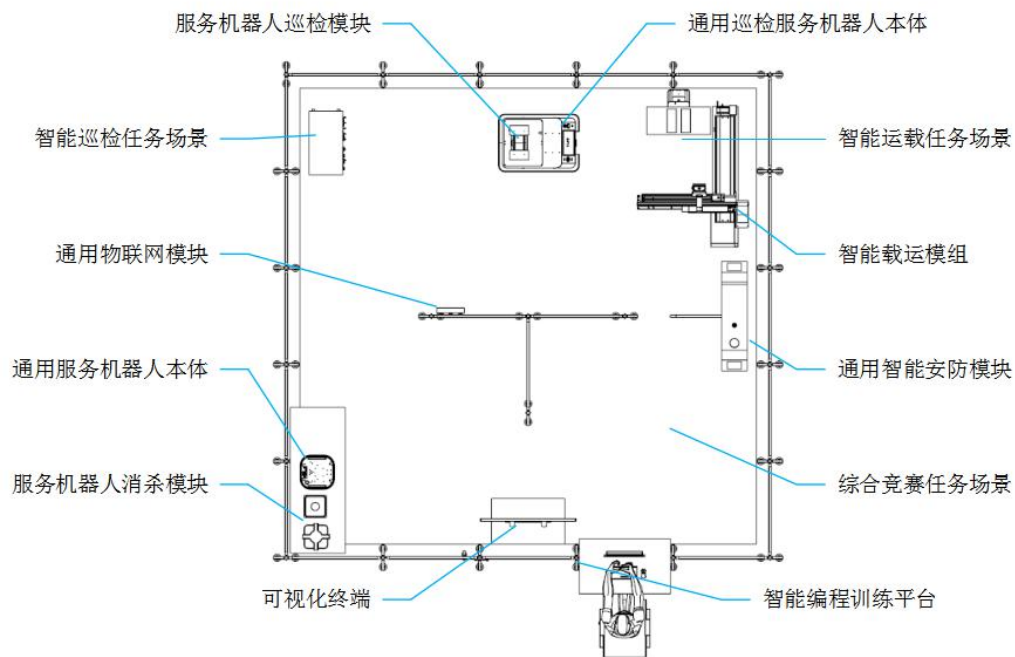
图 2 服务机器人人工智能技术应用平台俯视图（职工组）
