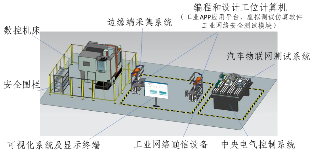
图 1 智能制造数字技术应用平台总布局简图
