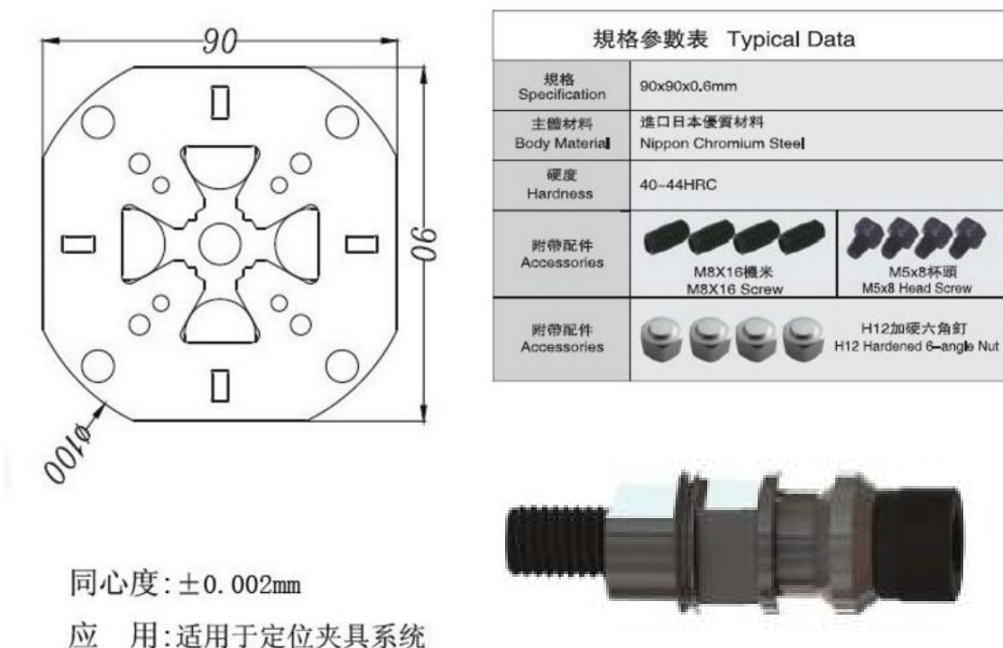
图5 方料治具定位片与拉钉
