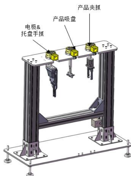
图 10 机器人快换夹具工作台示意图
